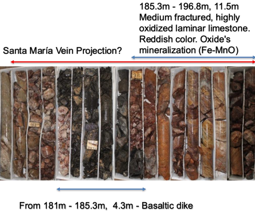
Foto 3 - Bohrkern SM20-42
