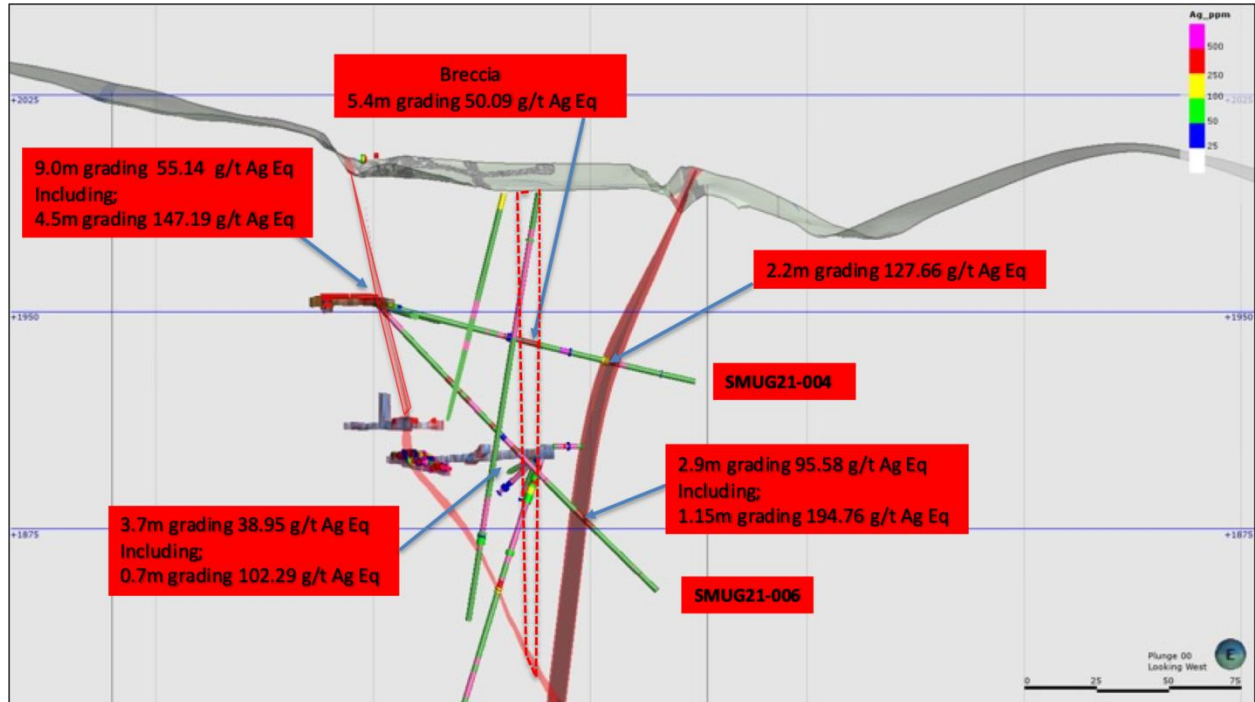
Abbildung 2 - Querschnitt der Bohrlöcher SMUG21-04, 06
