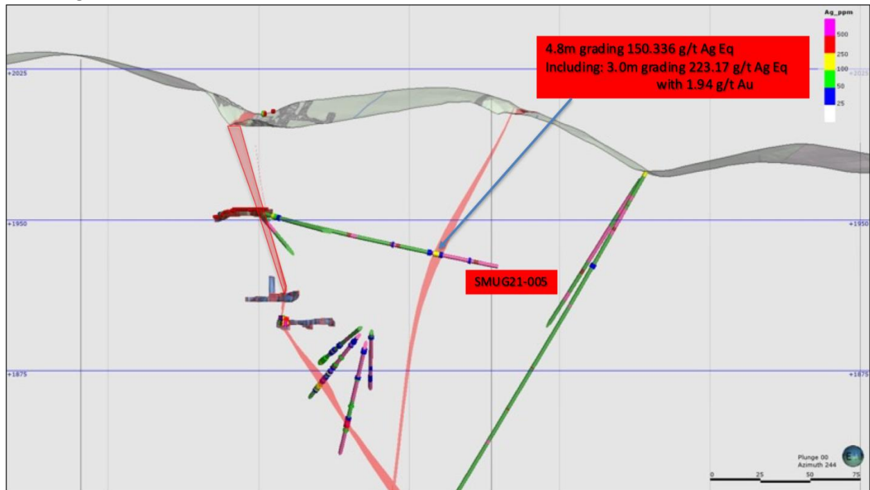
Abbildung 3 - Querschnitt von Bohrloch SMUG21-05
