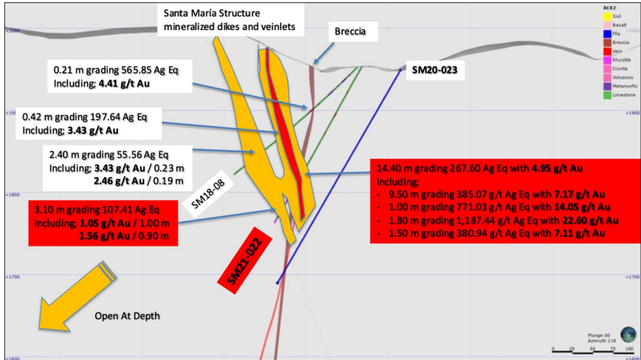
Abbildung 3 - Querschnitt von Bohrloch SM20-22
