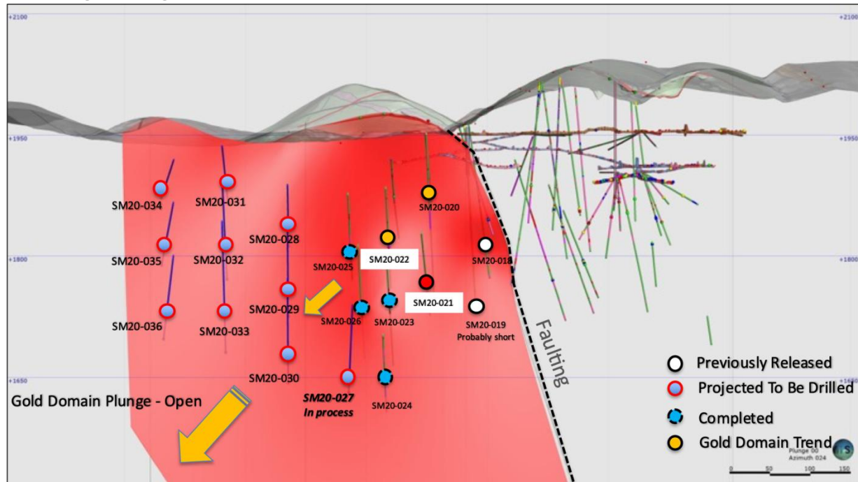
Abbildung 4 - Längsschnitt der Neuinterpretation
