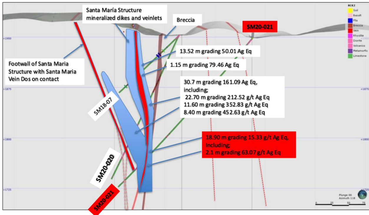
Abbildung 2 - Querschnitt von Bohrloch SM20-21
