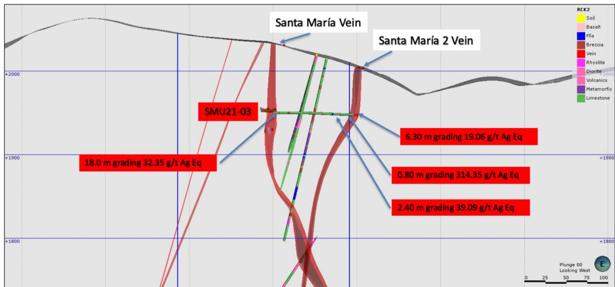
Darstellung 4 – Querschnitt der Bohrlöcher SMUG21-03
