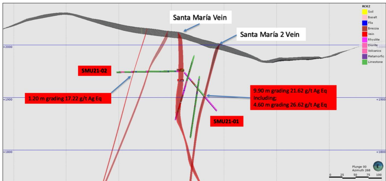
Darstellung 3 – Querschnitt der Bohrlöcher SMUG21-01, 02
