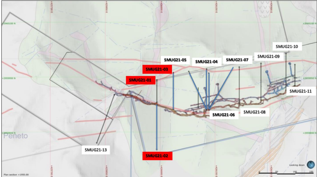
Darstellung 1 - Draufsicht des Gebietes der aktuellen Untertagediamantbohrungen
