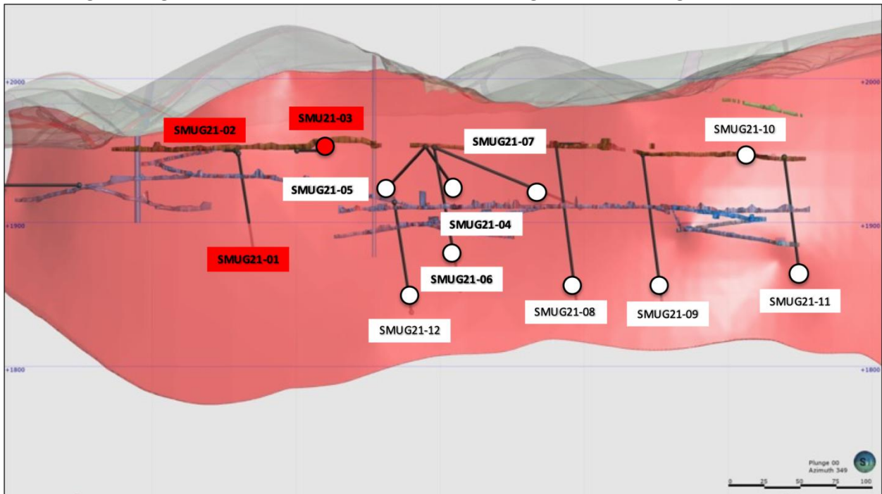
Darstellung 2 - Längsschnitt des Gebietes der aktuellen Untertagediamantbohrungen
